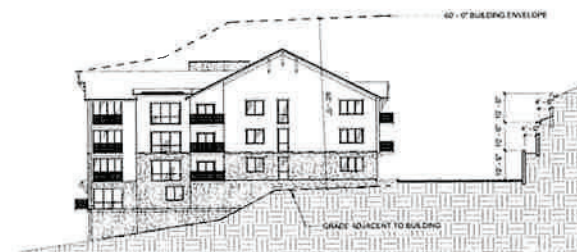
A3 SITE SECTION 1" = 20'-0"
